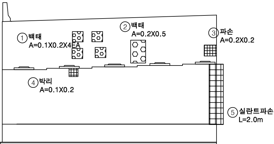
정면
