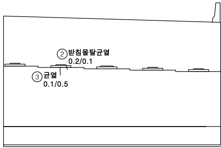
정면
