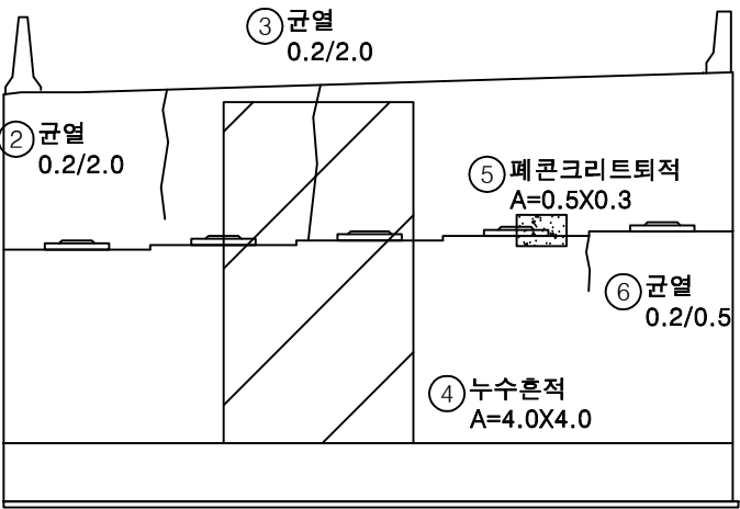
정면
